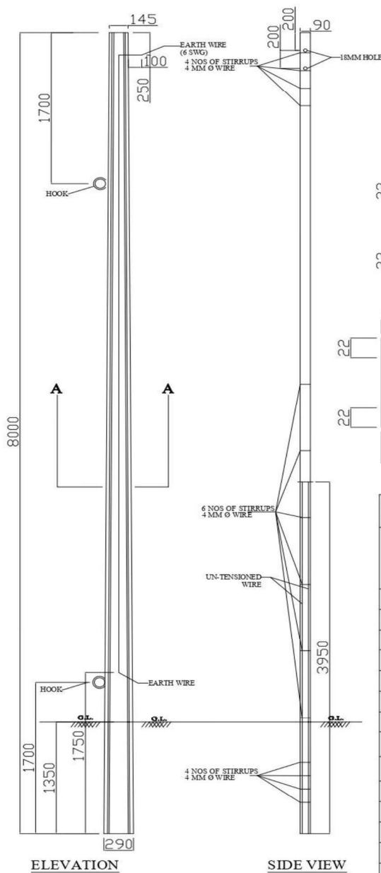
ELEVATION
